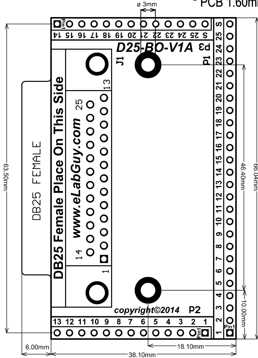
D25-BO-V1A PCB outline Drawing
