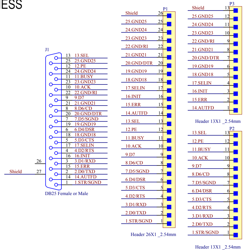
D25-BO-V1A Schematic Diagram
